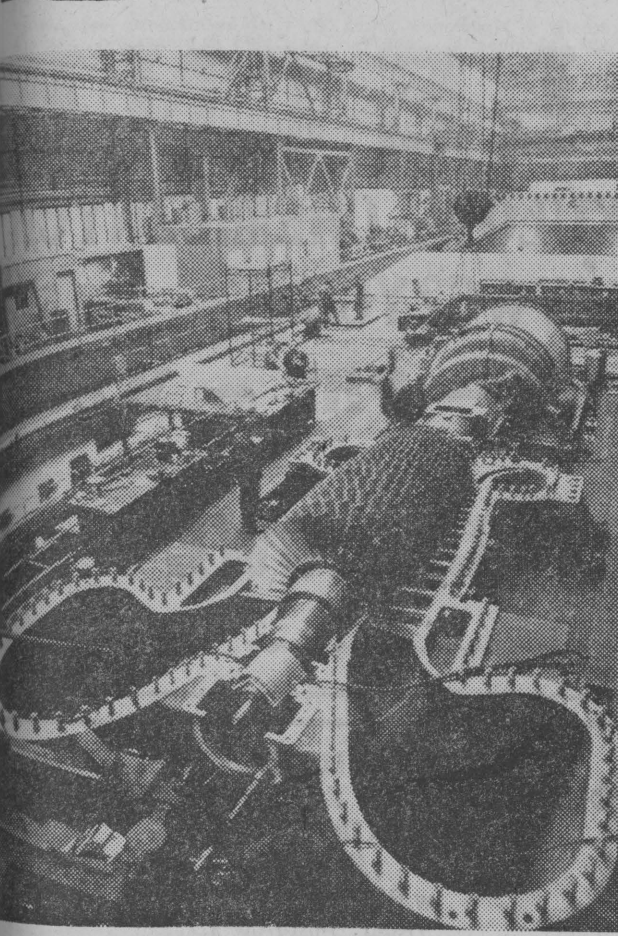
CSRS. Montaży turbospółki gigantycznego turbokompresora wyprodukowanego w zakładach mechanicznych w Pradze; jest on przeznaczony dla Związku Radzieckiego.
