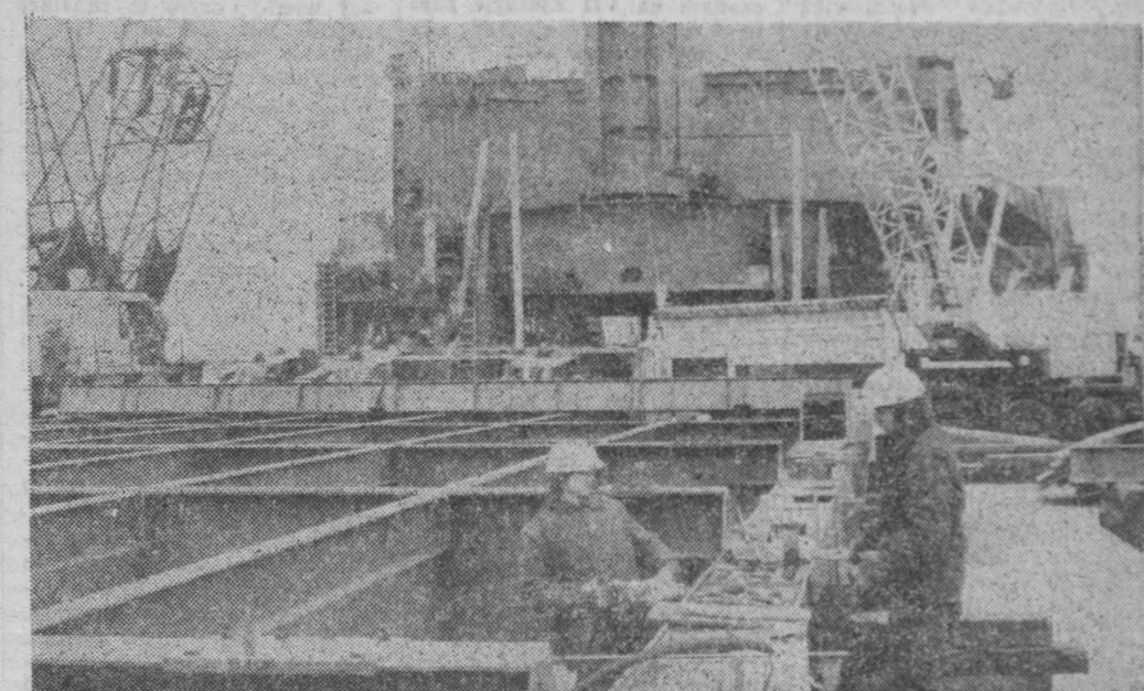
Od 15 października 1975 roku trwa budowa gigantycznej koparki kołowo-czerpakowej przeznaczonej dla kopalni węgla brunatnego Bełchatów. Po zakończeniu budowy 74-metrowa koparka ważyć będzie 7.120 ton, a jej wydajność wyniesie 110 tys. m. sześć. nakładu na dobę. Generalnym wykonawcą tej inwestycji jest warszawski „Mostostal”. NA ZDJĘCIU: budowa koparki. CAF — Zbraniecki
