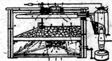
Rys. 4. Przekrój legnika. Strzałki wskazują ruch powietrza. Nad jajami widać termostat.
