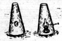
Rys. 5. Prześwitlacz do jaj można zrobić w domu z niezbyt grubej tekturki zwiniętej jak na rysunku i zszytej. Po zrównaniu dołu aby można było postawić przewietlacz nad lampą kuchenną, wycina się w nim otwór na wysokości płomienia lampy.
