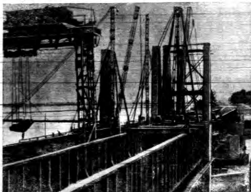
W przeciągu roku ukończona zostanie grobla łącząca wyspę Rungen z lądem stałym. Na zdjęciu technologiczne urządzenia budowlane.
