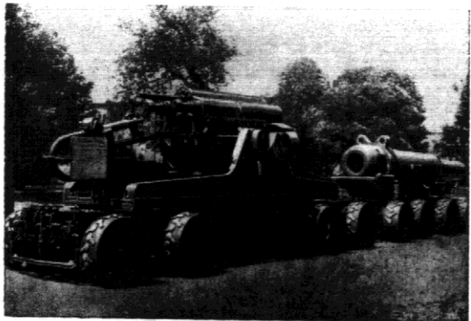
83 cm. hambina austriacka, która stała dotąd przed „Wiener Museum”, przewieziona została do Burgu „Grube Berta” wagi 51,700 kg., a maszyn jej wynosi 25 km.
