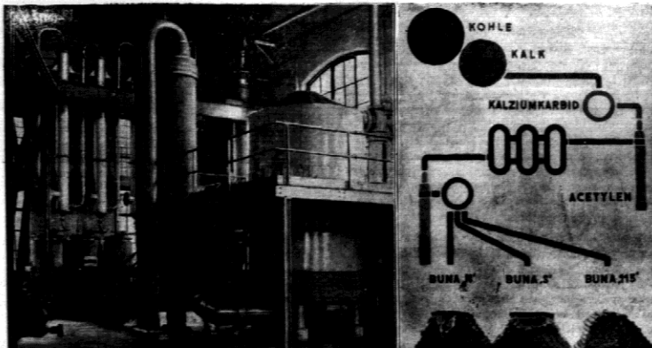
W Niemczech zaprowadzono syntetyczny kauczuk na wystawie samochodowej Urzędnictwa fabryczne wytwórni. Na prawo graficzne przedstawienie procesu.
