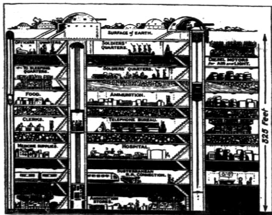
Kosztom wielu miliardów wybudowała Francja, w latach powojennych, wzdłuż całej swej granicy wschodniej, fortyfikacje podziemne. Na zdjęciu plan takiego fortu, sięgającego na 325 stóp w głąb.
