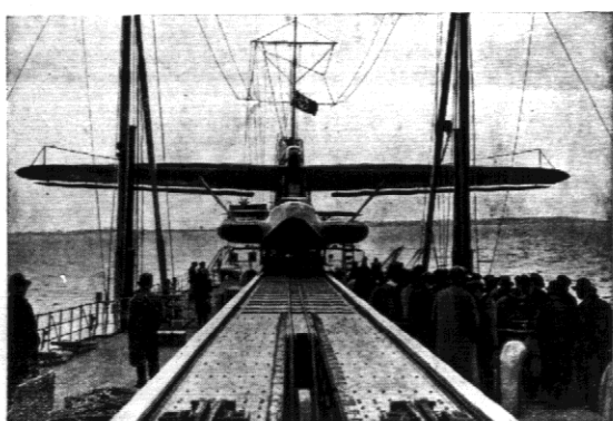
Parowiec „Ostmark” z urządzeniem katapultowym dla samolotów.
