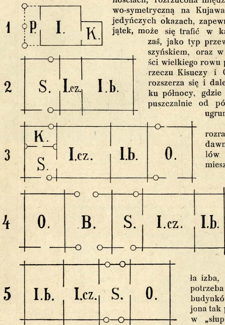
Rys. 127. Rozwój chaty jednoizbowej. (Podług L. Puszczy. I. b = izba biała. I. cz. = izba czarna. S. = sień. K. = komora. O. = obora (stajnia). B. = boisko (klepisko) z siankami. P. = podcienie.
