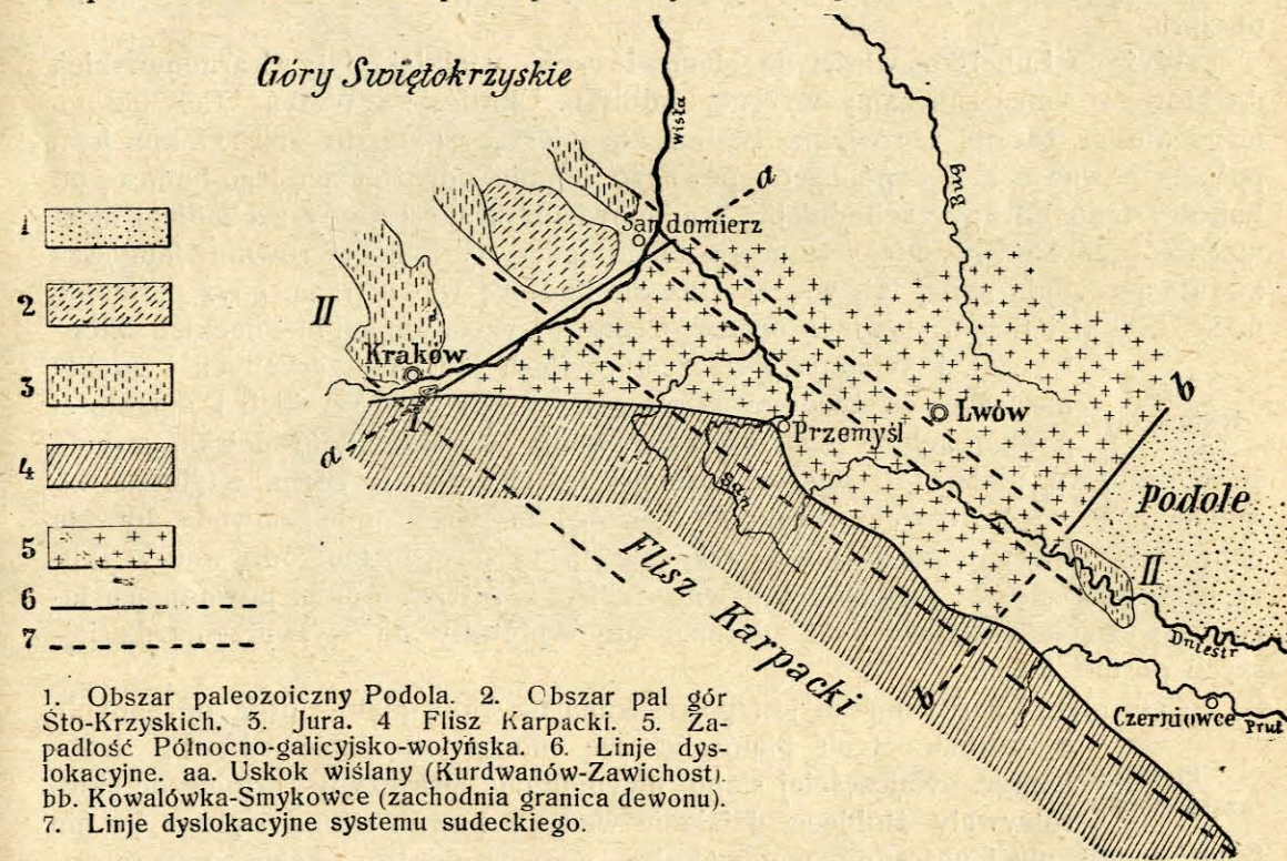
Rys. 48. Schemat tektoniki zapadłości podkarpackiej. (Podl. Tesseyre'a).
