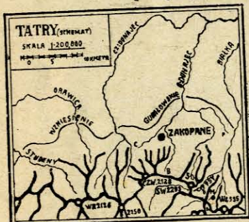
Rys. 21. Schemat rozgałęzienia Tatr. (Podl. O. Sosnowskiego).
