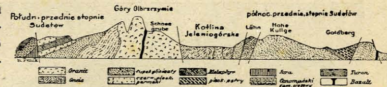
Rys. 2. Przekrój przez Góry Olbrzymie. (Podług G. Güricha).
