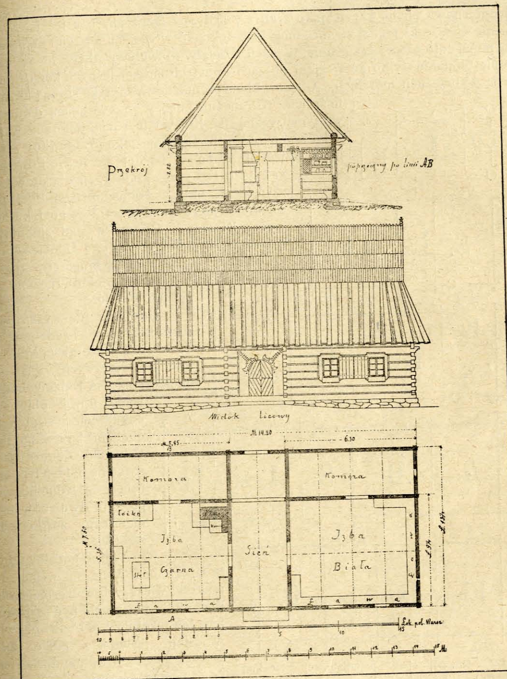
Rys. 126. Chałupa dwuizbowo-symetryczna na Podhalu.
