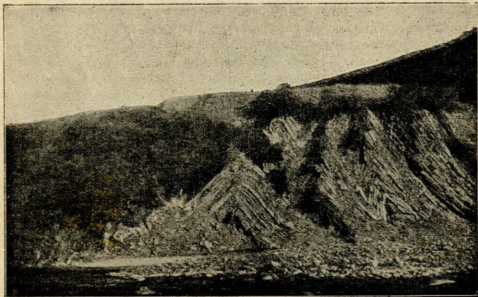
Rys. 17. Fałdy piaskowcowe w dolinie Prutu. (Podł. prof. Szajnochy).
