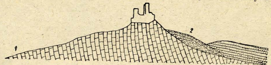
Rys. 44. Schemat budowy geologicznej góry Zamkowej w Chęcinach. (jedna część antyklinali podług Sobolewa).
