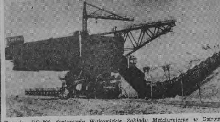
Koparkę DO-800 dostarczyły Witkowskie Zakłady Metalurgiczne w Ostrowie dla Kopalni siarki w Piasteczku (na zdjęciu).
