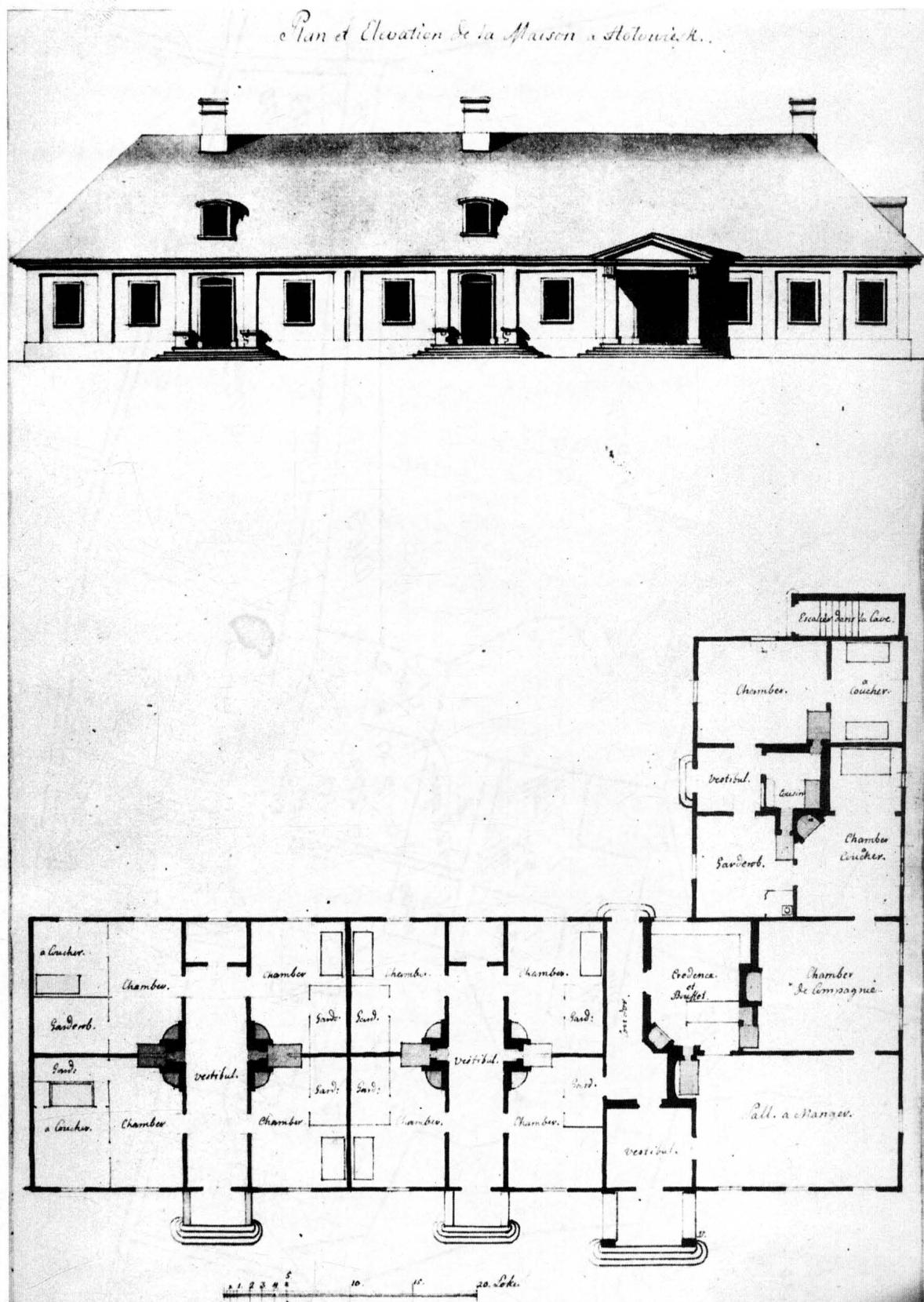
38. Bielsk Podlaski, gm. Bielsk Podlaski. Hołowiesk. Dwór - elewacja główna i rzut poziomy na nieistniejącym dziś rysunku (do 1944 r. przechowywanym w BUW, Gabinet Rycin, Zbiory Króla Poniatowskiego 187, nr 180 zatytułowanym „Plan et Elevation de la Maison a Hołowiesk”). Fotokopia sprzed 1939 r. ODZ Warszawa, Teki Glinki, 235 fot. 34. Neg. OW PSOZ Białystok nr D 2517.
