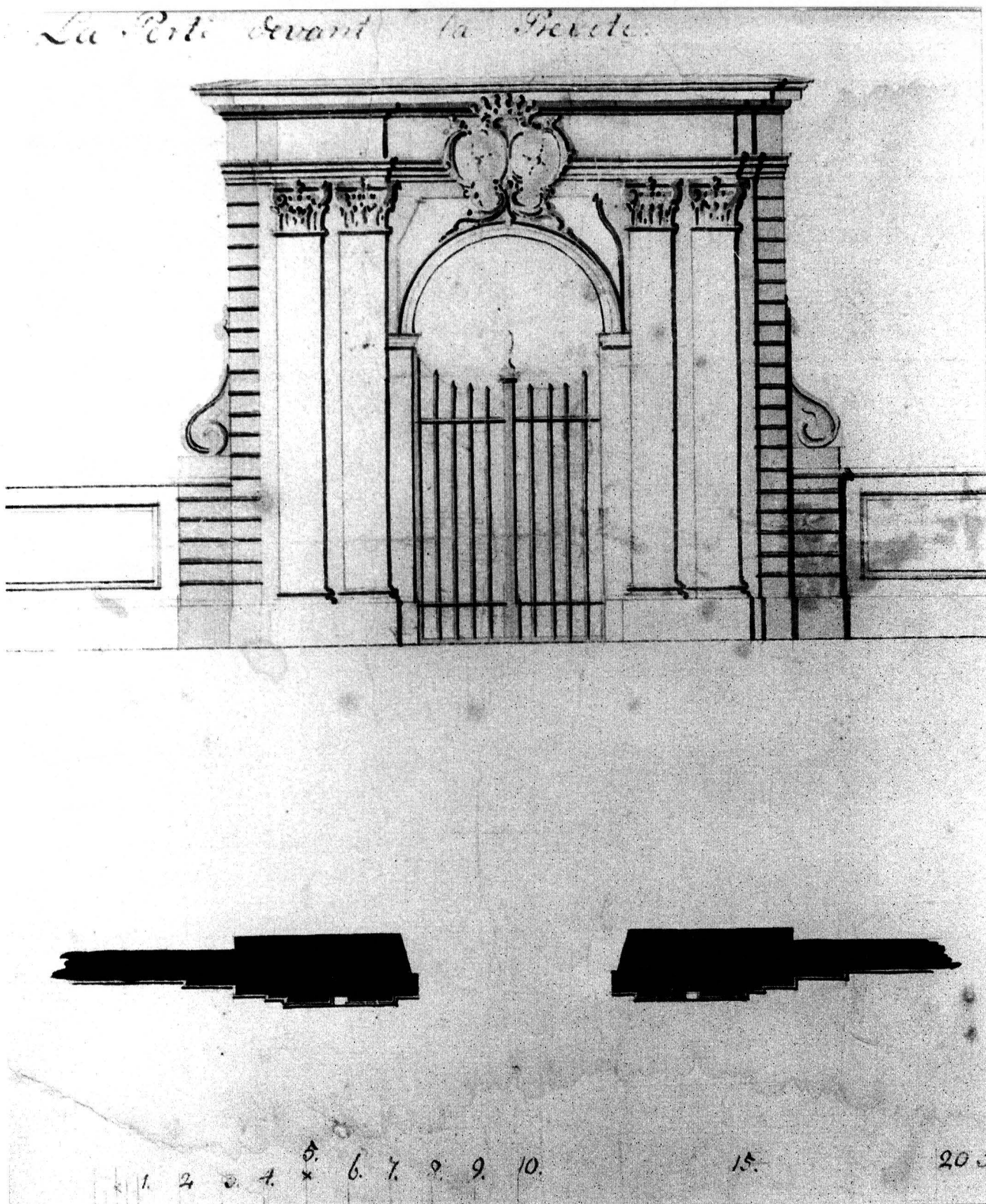
35. Białystok. Ogród Bartolomitów przy probostwie kościoła farnego. Brama przed plebanią - rzut i elewacja. Projekt wyk. ok. poł. XVIII w. - „La porte devant la Preveté”. BUW, Gabinet Rycin, Zbiory Króla Poniatowskiego nr 187, nr 137. Neg. OW PSOZ Białystok nr D 2727.
