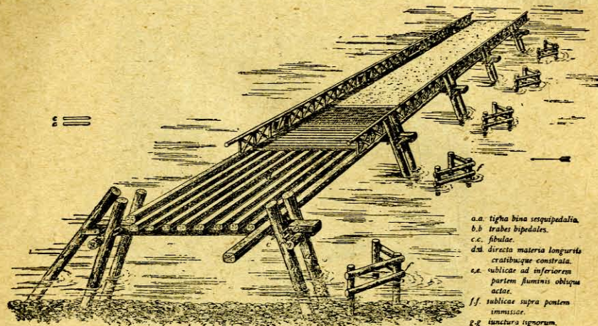
Most Cezara.
