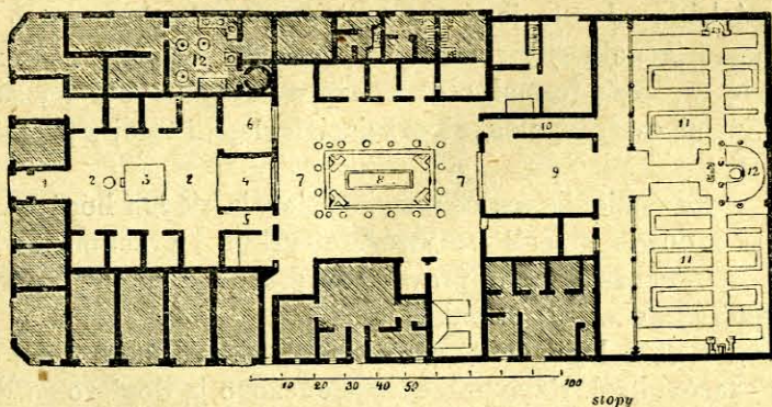
Plan domu.
