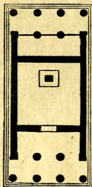
Amfiprostyl.
