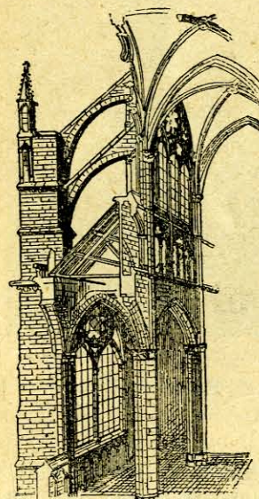
Przekrój konstrukcji gotyckiej.
