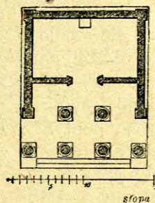
Plan świątyni tuskańskiej.
