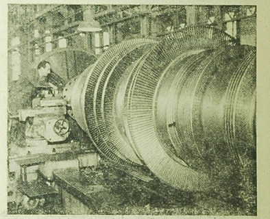
NA ZDJĘCIU: montaż potężnego wirnika do turbiny o mocy 125 MW, jaką obłaski „Zamech” dostarczył stołowiejskiej elektrowni Trbovlje.
