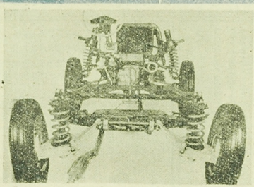
Podwozie nowego typu samochodu „Wartburg” widziane od tyłu. Ten nowy typ znanego u nas samochodu fabryki w Eisenach (NRD) posiada silnik 3-cylindrowy, dwukrotny pojemności 691 cm sześci, o mocy 45 KM przy 2700 obr. na minutę. Sztywność nadk. — 120 km/godz. Zużycie benzyny 8,5 do 9,5 l/100 km.
