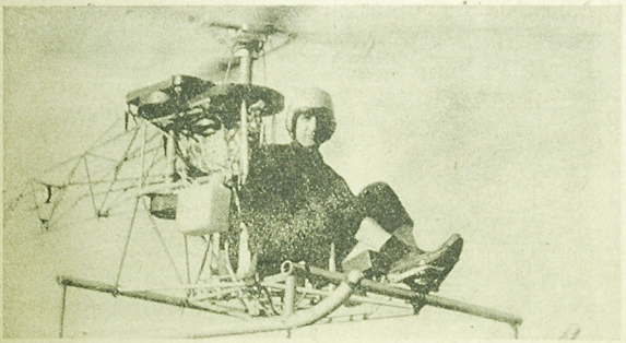
Bestwloczenie Genewy M. Starczaka na Helikopterze własnej konstrukcji. Helikopter wykonany jest głównie z części samochodu marki „Wolkswagen”.
