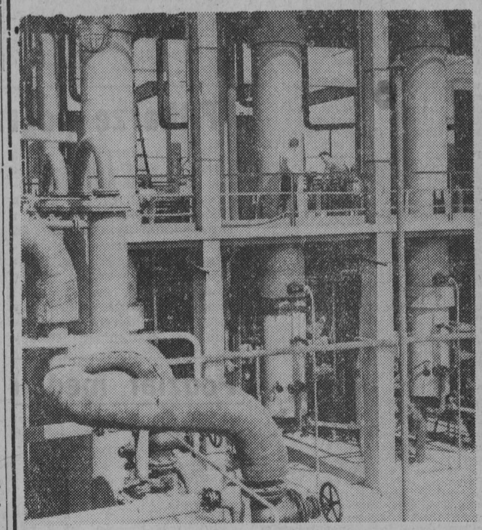
W dniu 29. VIII. 1960 r. w Zakładach Azotowych im. F. Dzierżyńskiego w Tarnowie nastąpił próbny rozruch oddziału cykloheksanolu służącego do produkcji kaprolaktamu — podstawowego surowca przy produkcji włókien sztucznych. NA ZDJĘCIU: fragment nowego oddziału. CAF — fot. Grzęda
