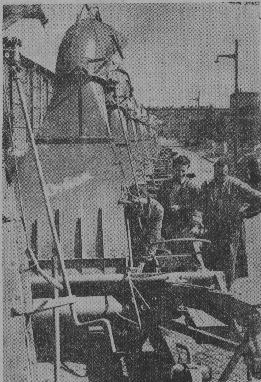
Poznańska Fabryka Maszyn Zróżnicowanych rozpoczęła w czerwcu br. produkcję ścinaczki zielonek „Orkan”. Jest to nowoczesna maszyna uniwersalna o prostej a jednocześnie silnej konstrukcji. Służy do ścinania zielonek zarówno niskich (trawa, lucerna, lubin) jak i wysokich (mieszanka itp.), przeznaczonych do spasania „Orkanów”, do silosowania. W roku bieżącym poznańska fabryka opuści 500 sztuk „Orkanów”. NA ZDJĘCIU: ostatnia kontrola techniczna wyprodukowanych ścinaczek zielonek „Orkan”.
