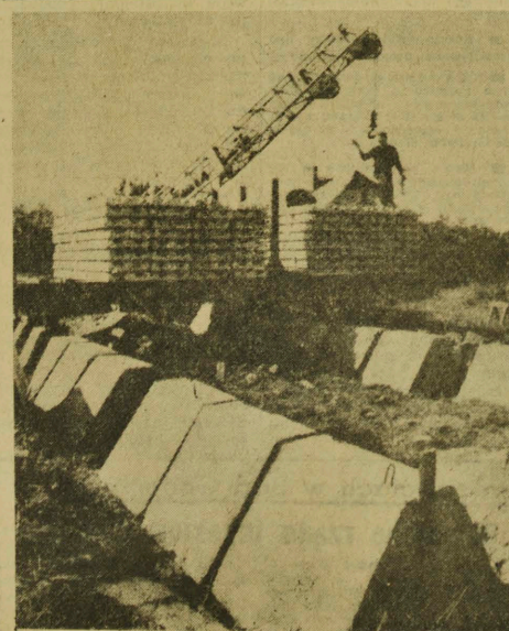
W południowej Czechosłowacji buduje się domy prefabrykowane nowego typu. Nowa metoda polega na układaniu bloków fundamentu w matych odległościach od siebie. Dzięki wprowadzeniu nowej metody oszczędza się 20 — 30 proc. betonu i 30 — 40 proc. stali.
