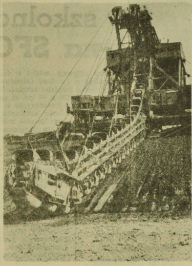
Dobiegają końca prace przy budowie największej kopalni rejonu Konina — odkrywkę węgla brunatnego „Pątnów”. Uruchamiana kopalnia „Pątnów” dostarczać będzie paliwo do pobliskiej elektrowni „Konin”. Jej docelowe wydobycie — 3.700 tys. ton węgla rocznie — osiągnięte zostanie w najbliższych latach.
