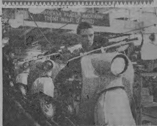
Mija już drugi miesiąc jak w Warszawskiej Fabryce Motocykli ruszyła druga taśma montażowa przeznaczona wyłącznie do produkcji skutera „Osa”. Do tego czasu „Osa” była składana na przemian z WFM-ką pasażerską; jednego dnia skuter „Osa”, drugiego — motocykl WFM. Dzięki nowej taśmie, jeszcze w tym roku miłośnicy motoryzacji otrzymają 6500 skuterów. NA ZDJĘCIU: nowa taśma „Osa”. Na pierwszym planie przy pracy monter B. Świadek.
