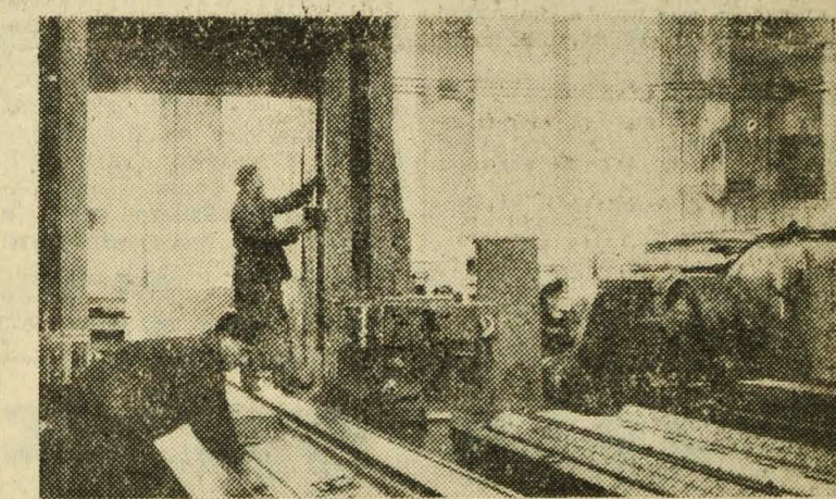
Fabryka Urządzeń Mechanicznych „Poreba” w Porebie produkuje wyłącznie ciężkie obrabiarki do metali. Ten stary, liczący już ponad 160 lat zakład, znajdujący się w stałej rozbudowie, około 40 proc. swojej produkcji przelicza na eksport. NA ZDJĘCIU: fragment montażu CAF — fot. Kondracki
