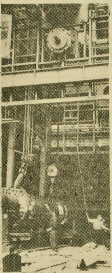
1 listopada br. w budującej się elektrowni na Siekierkach w Warszawie zostanie oddany do użytku pierwszy turbozespół o mocy 50 megawatów. NA ZDJĘCIU: potężny kocioł o wadze 42 ton na chwilę przed wciągnięciem na konstrukcję. CAF — fot. Uchymiak
