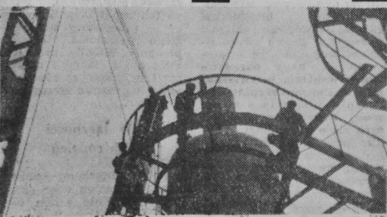
NA ZDJĘCIU: fragmenty montażu urządzeń do ciągłej produkcji paku utwardzonego w Zakładach Kokso-Chemicznych „Blachownia”. CAF — fot. Seko
