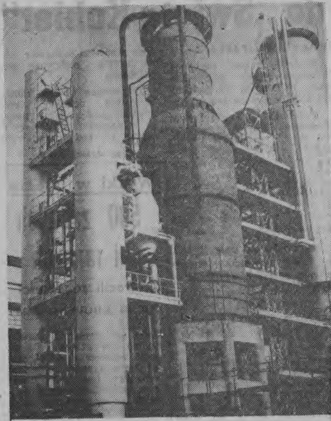
Fragment aparatury destylacyjnej kombinatu chemicznego „Slovaft” w Bratysławie. FOT. - CAF
