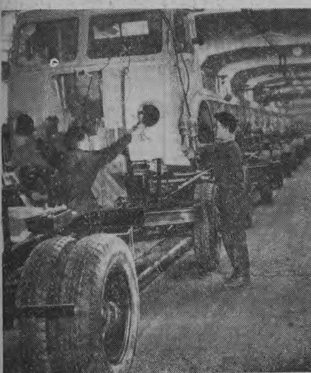
Najbardziej znanym w naszym kraju samochodem ciężarowym jest „Star” — produkcji Fabryki Samochodów Ciężarowych w Starachowicach. Czołowy ten zakład przemysłu motoryzacyjnego już niedługo przejdzie na produkcję samochodów zapędzonych w silnik wysokoprężny polskiej konstrukcji, w miejsce mniej ekonomicznego benzynowego. NA ZDJĘCIU: montaż „Starów” na taśmie. CAF — fot. Czarnogórski
