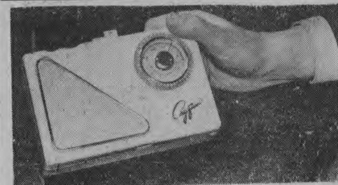
Nowy tranzystorowy odbiornik radiowy — Illput na długie i średnie fale, o wadze 850 gramów i wymiarach 185x125x48 mm. Prąd do odbiornika dostarcza cynkowy-kadmowy akumulator oraz bateria słoneczna.
