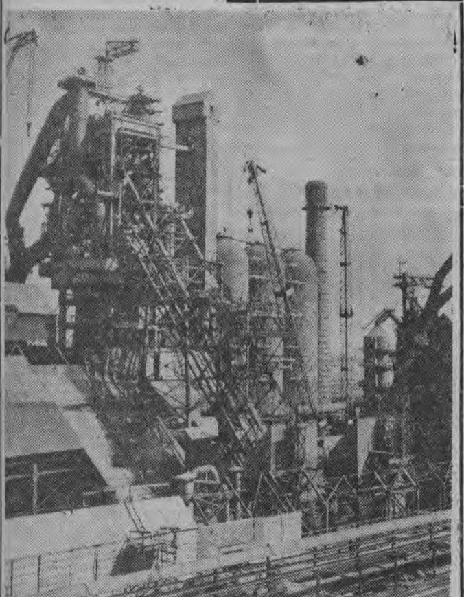
Za niecałe 3 miesiące ruszy wielki piec nr 3 w hucie im. Lenina. Jest to największy w Polsce piec hutniczy. NA ZDJĘCIU: fragment budowy 3-go wielkiego pieca. Fot. — CAF
