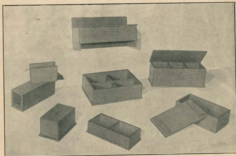
Modele: pudełko wiszące, pudełko na przezrocza (na powtórzenie ćwiczeń), szkatułka (ćwicz. 1, 2, 3, 15 i 16), skarbonka, pułapka na myszy (na powtórz. ćwicz.), pudełko z przegródką na drobiazgi (ćwicz. 1, 2, 3, 5 i 15), pudełko na gwoździki (ćwicz. 1, 2, 3, 5, 15 i 17).
