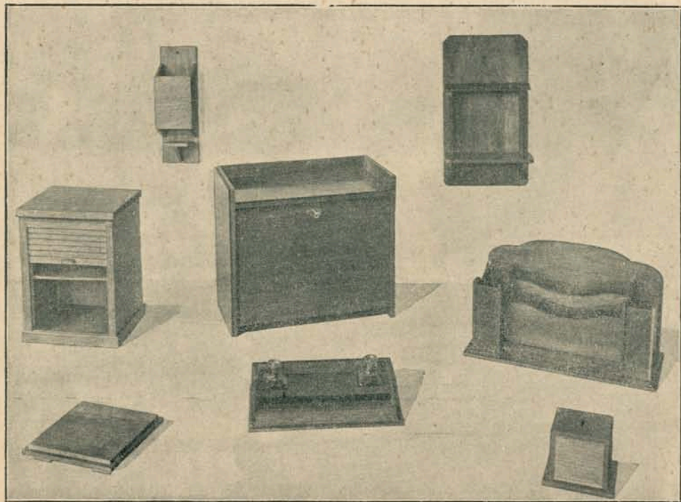
Modele na powtórzenie ćwiczeń: szafka z żaluzją, podstawka, kałamażnica, skarbonka, segregator, kasetka, pułeczka wisząca na zapalki, pułeczka wisząca na kredę.
