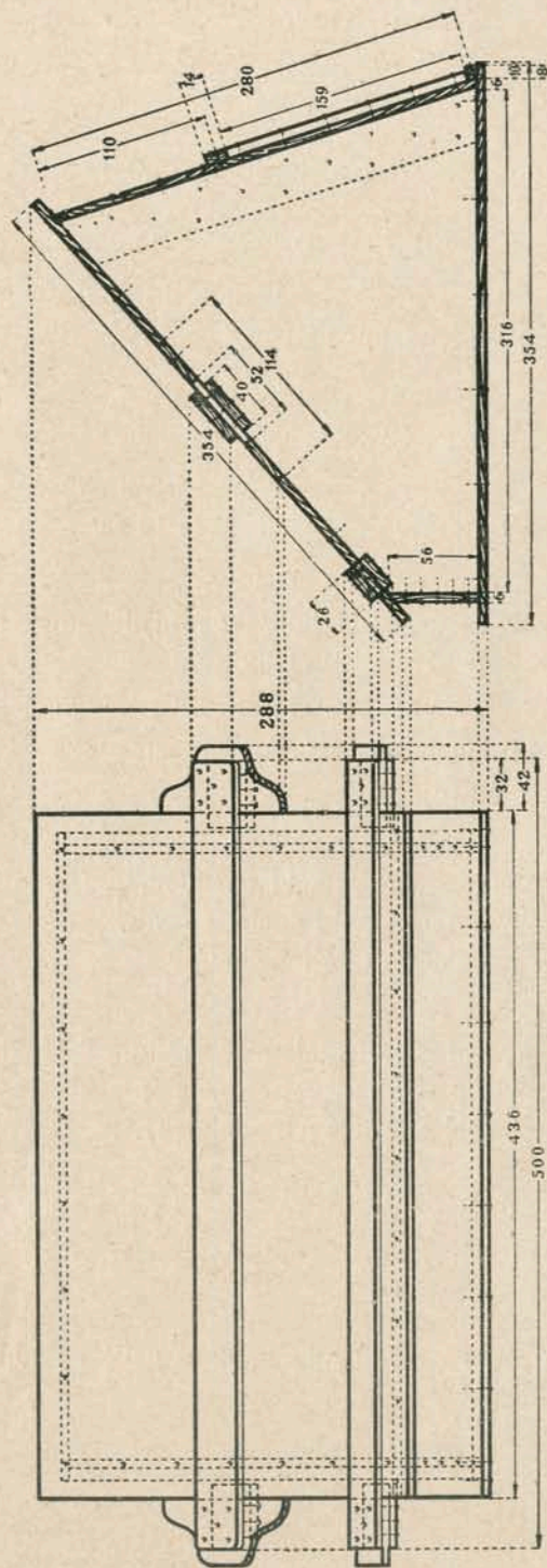
RYS. 18 c PULPIT DO PISANIA GRAFICZNEGO
