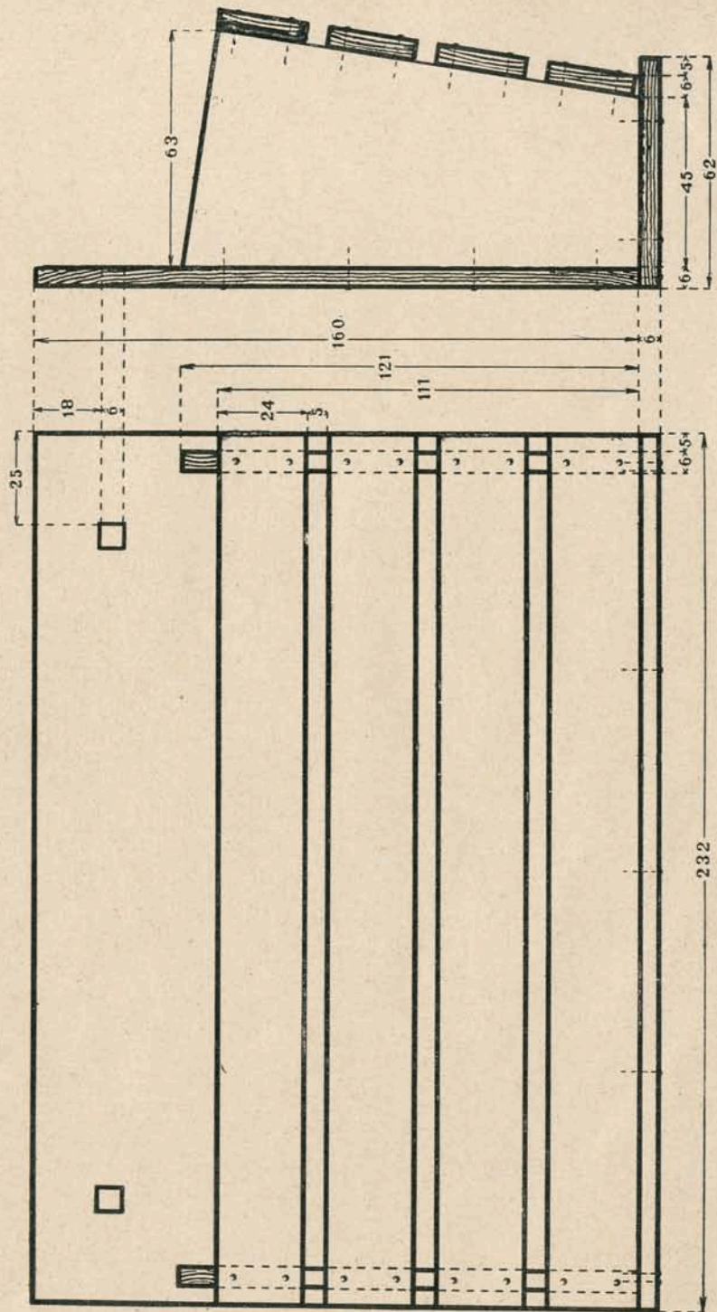
RYS. 13 b . PUDEŁKO WISZĄCE NA LISTY
