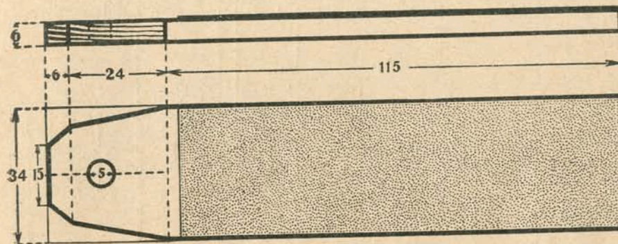
RYS. 7 a . DESECZKA DO OSTRZENIA OŁÓWKÓW
