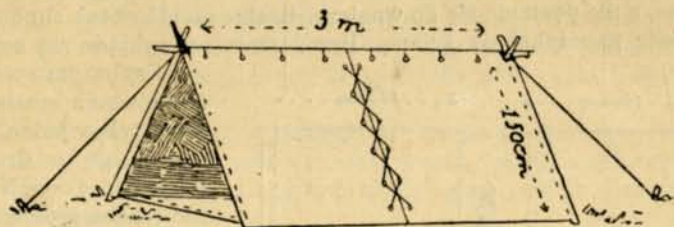
Namiot dla jednego patrolu. Cztery płótna tworzą ściany, dwa — postanie.
