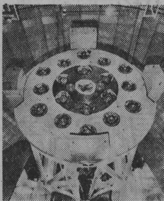
Drugi co do wielkości na świecie teleskop, który służył do obserwacji sztucznych satelitów ziemskich w czasie Międzynarodowego Roku Geofizycznego. Teleskop znajduje się w Obserwatorium Lick w Kalifornii (USA) ma 120 cali średnicy, a wykonanie jego soczewki trwało 10 lat.
