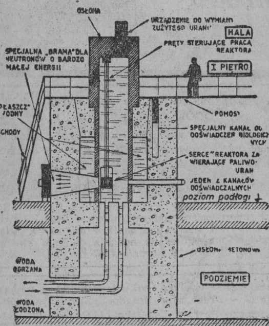
Oto reaktor w przekroju pionowym
