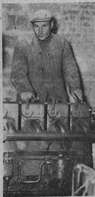
Tzw. główna „siłownia” Mielnickich Zakładów. 48-konny motor Diesla i jego opiekun Antoni Kierkowski. Fot. „Gazeta” — Z. Z.
