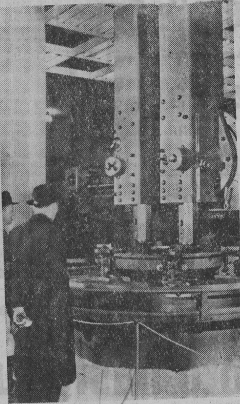
W pawilonie polskim. Tokarka karuzelowa, model 2,5 KBE-R. Główny silnik napędowy posiada moc 22 Kw. (największa średnica obrabianego przedmiotu wynosi 2100 mm, maksymalna wysokość obrabianego przedmiotu — 450 mm). Fot. — CAF
