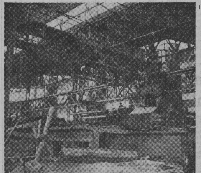
Budowa największej w Europie walcowni blach ciągłych na gorąco w Hucie im. Lenina postępuje szybko naprzód. NA ZDJĘCIU: fragment budowy hali i montażu urządzeń dostarczonych przez Związek Radziecki. Fot. — CAF
