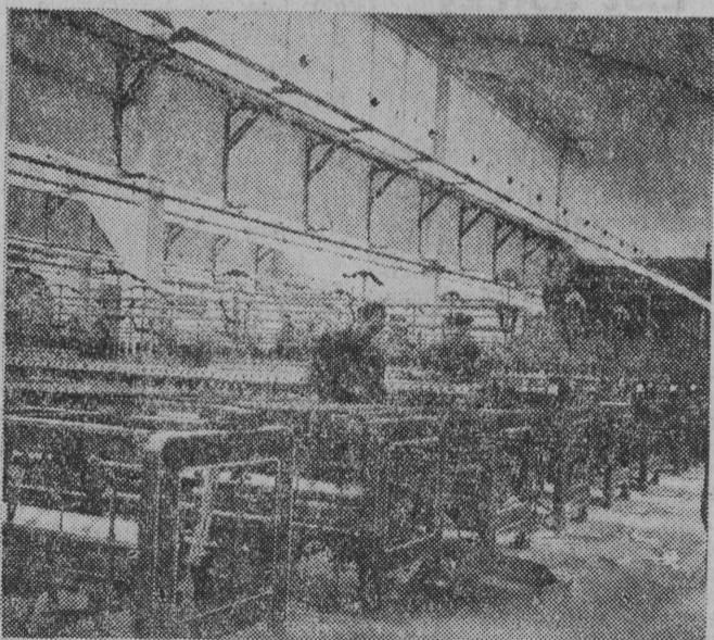
W nowej przedalni przy Zakładach Przemysłu Bawełnianego im. Armii Ludowej w Łodzi trwa montaż maszyn przędzalniczych.
