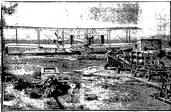
Technika dzisiejsza czyni wysiłki, aby start i lądowanie samolotów odbywało się na jaknajmniejszym terenie, wysiłki te zostały częściowo uwieńczone rezultatami dodatkami w stosunku do wodnioplawców, które startują z okrętów przy pomocy katapult. Ilustracja nasza przedstawia próbę zastosowania specjalnego podwozia z urządzeniem katapultowym przy samolocie lądowym.
