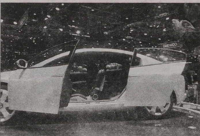
Ciekawa koncepcja konstruowania drzwi. Przednie otwierają się zupełnie konwencjonalnie, zaś tylne – „jadą” do tyłu. Środkowego słupka brak...
