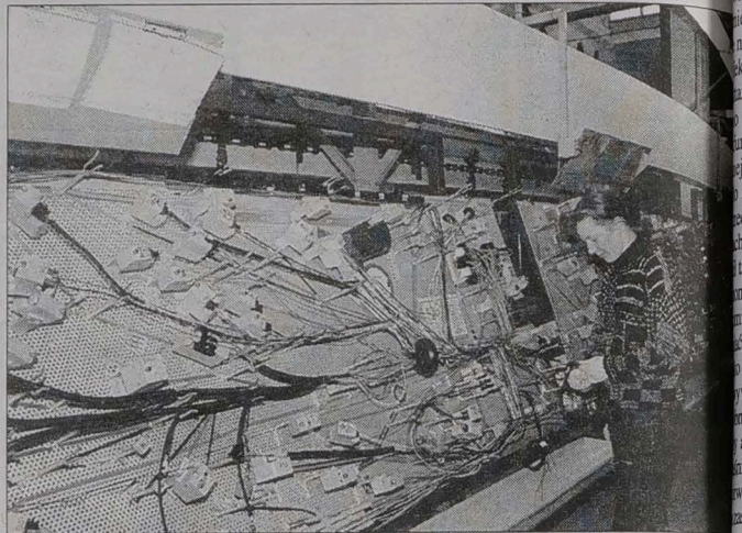
Montaż wiązki instalacji elektrycznej do FORDA Ka
