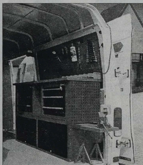
Przykład zagospodarowania warsztatu na kołach. Narzędzia na wieszakach i w specjalnie przygotowanych szufladach. Imadło na specjalnie wysuwającym blacie.
