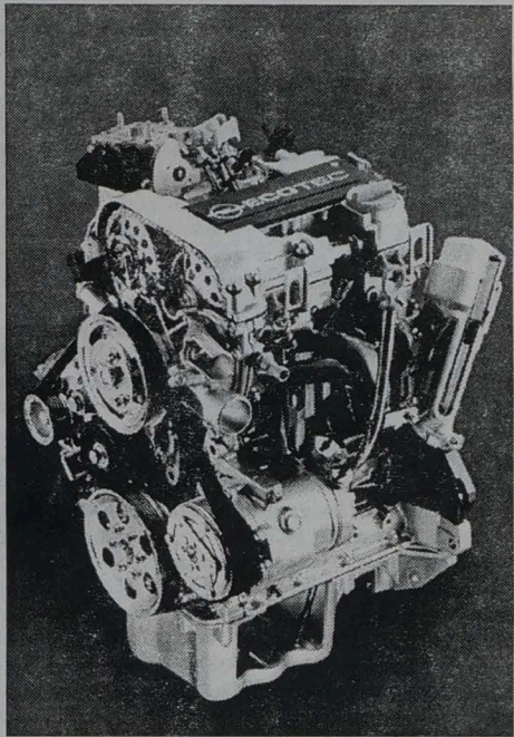
Trzycylindrowy silnik z rodziny ECOTEC zadziwia swoimi rozwiązaniami technicznymi i technologicznymi. Jest to bardzo nowoczesna jednostka napędowa.
