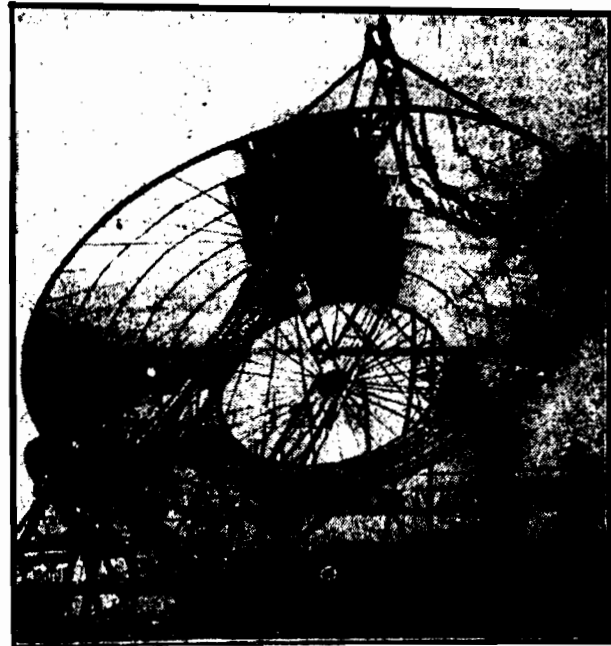
Oto maszyna parowa — duma Kalifornii — ze stalowym cylindrem, który mieści 800 litrów wody nagrzewanej promieniami słonecznymi. Maszyna obsługuje pompę, która tłoczy 5 tysięcy litrów wody na minutę.
