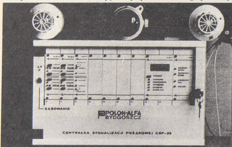
Centrala sygnalizacji pożarowej
