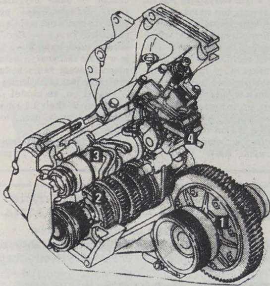
Skrzynia biegów nowej generacji, gwarantująca błyskawiczną zmianę biegów. 1 — mechanizm różnicowy napędu osi przedniej, 2 — zespół kół przekładni, 3 — wałek uruchamiający przekładnię, 4 — drążek zmiany przełożeń.
