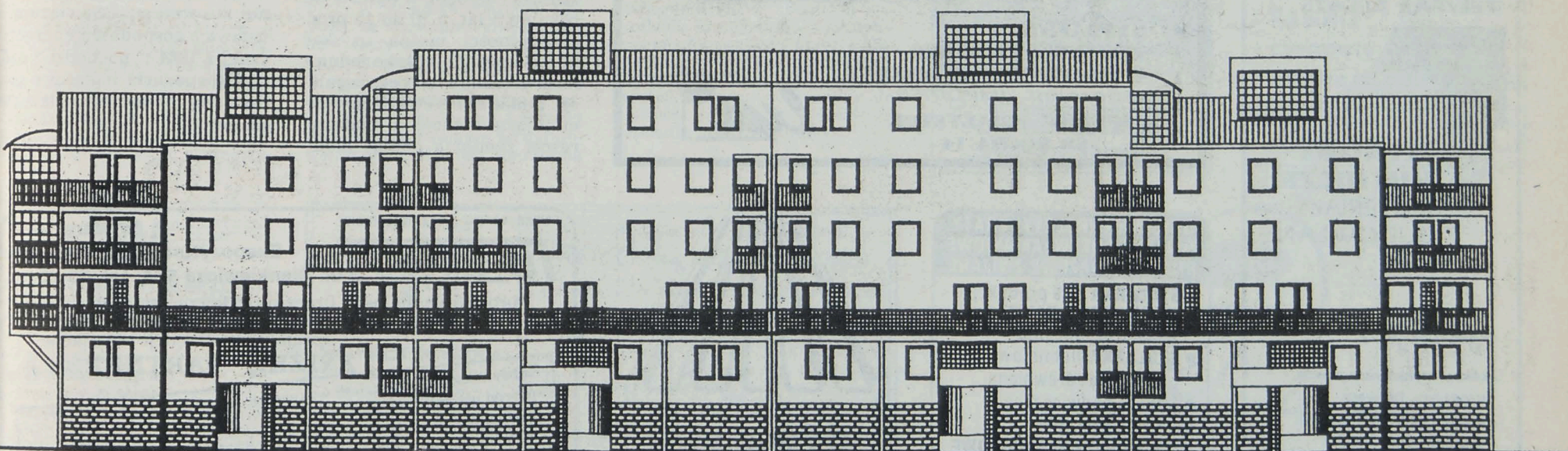
ELEWACJE 1:200
