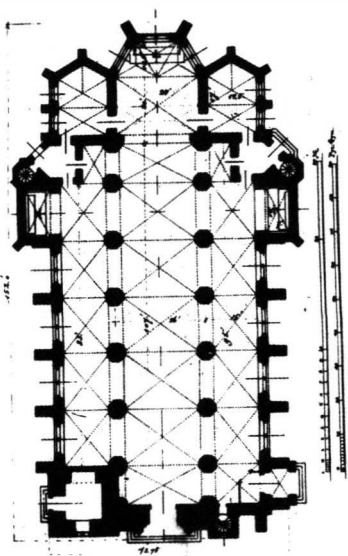
Poświętne. Rzut poziomy kościoła
