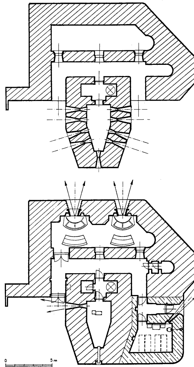
Blokhauz Nr 1024 przed przebudową (A) oraz jako tradytor artyleryjski sektora „Osowiec” (B)
