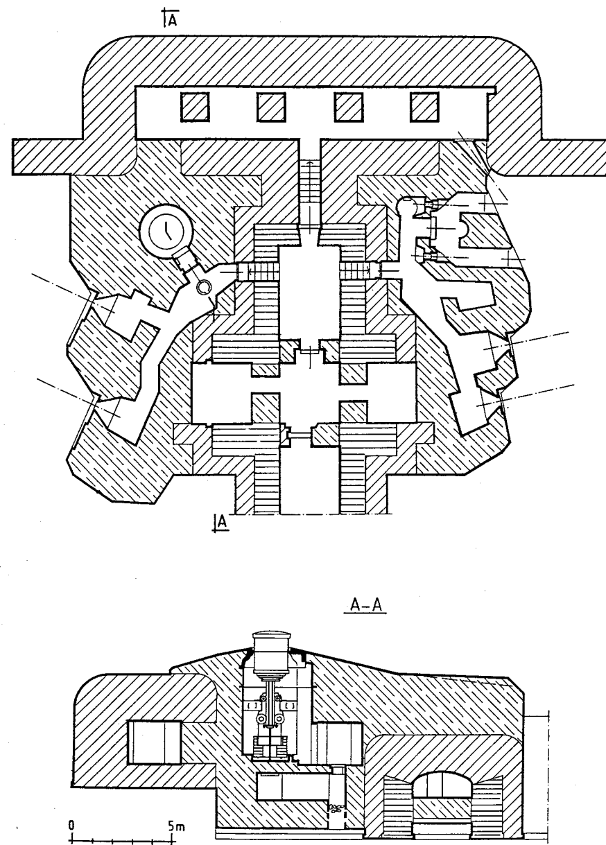
Obiekt nr 2 Fortu II
