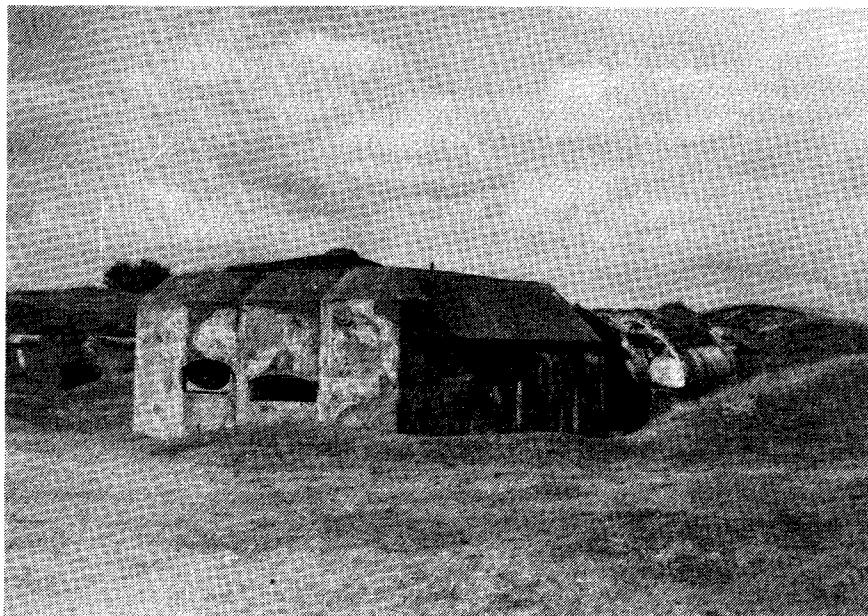
Obiekt nr 1 Fortu II. Widok z zapola
