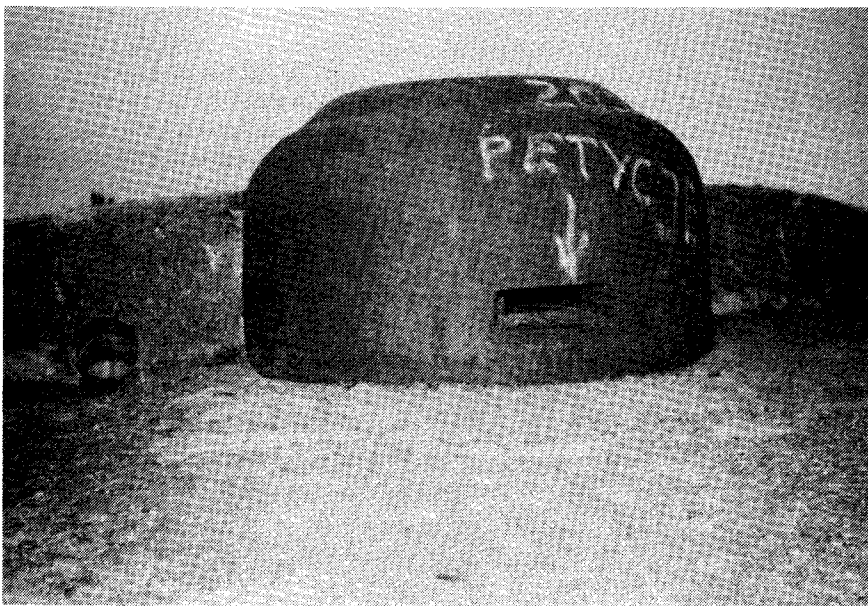
Pancerna półkopuła obserwacyjna obiektu nr 1
